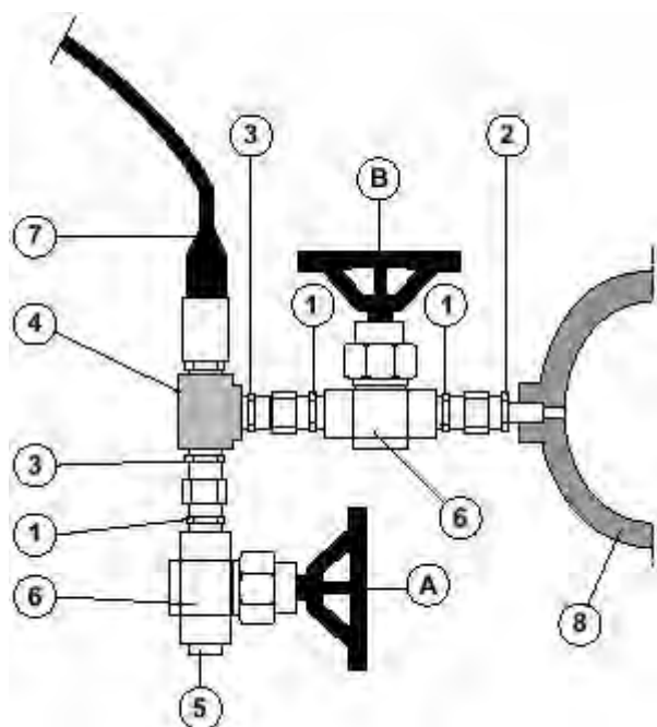
Рис. 10. Монтаж датчика давления при помощи монтажного комплекта
