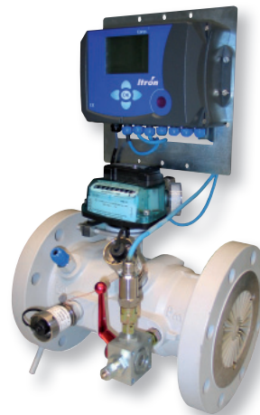
TZ|FLUXI с корректором объема газа CORUS
