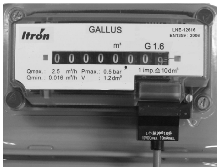
Рис. 2.5. НЧ датчик импульсов, смонтированный в гнездо отсчетного устройства счетчика
